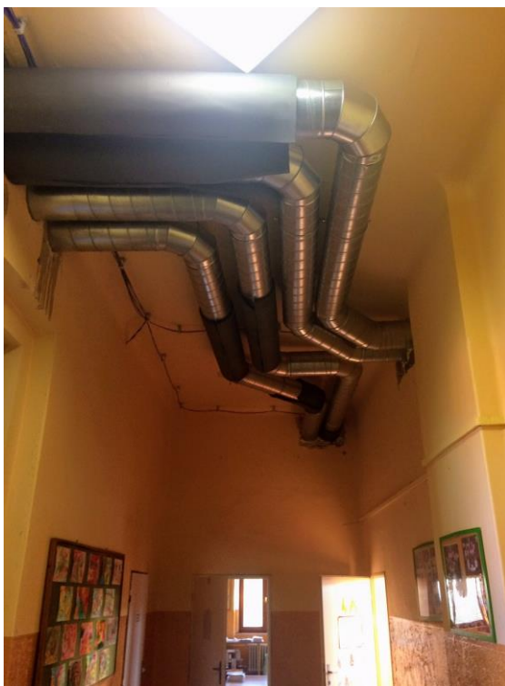
Ještě nezakryté rekuperační potrubí na chodbě a jednotka ve třídě č. 9
